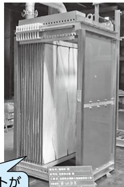
膜ユニット
