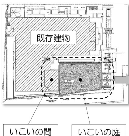
◀図書館本館配置図▶
