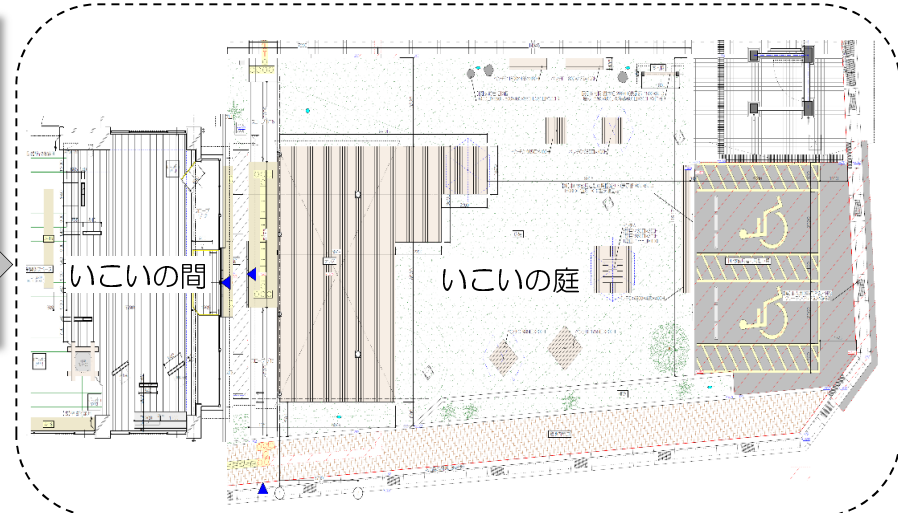
◀「いこいの間」「いこいの庭」平面図▶
