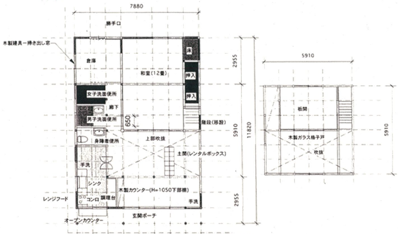
平面図
