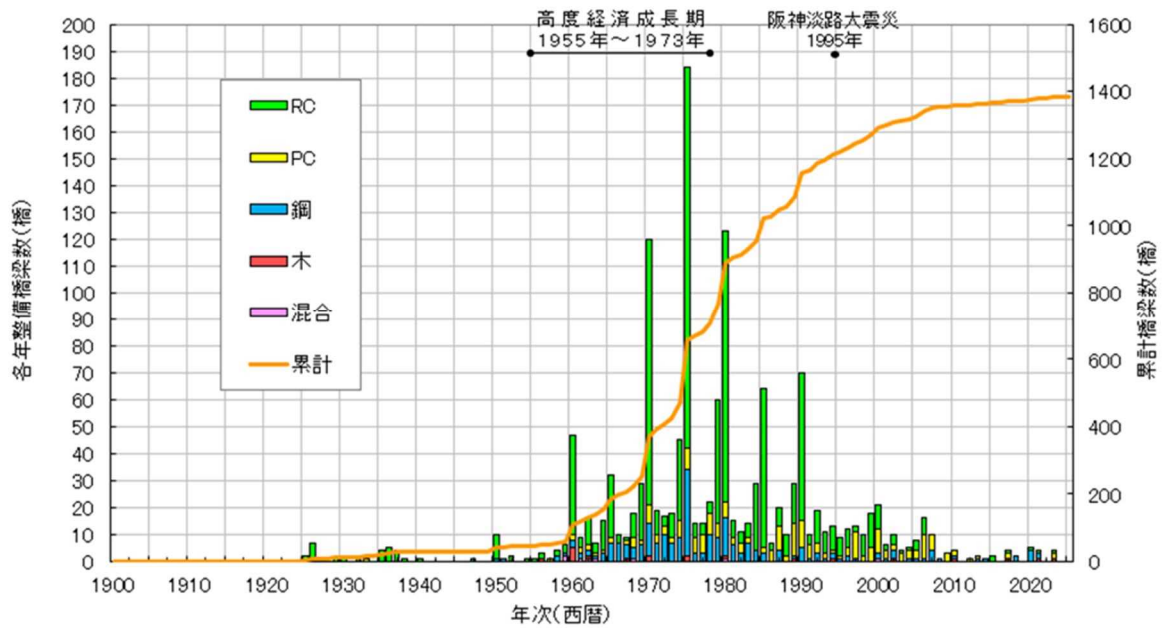
豊岡市が管理する橋梁の架設状況
