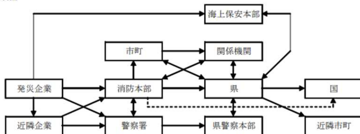
情報系統図
