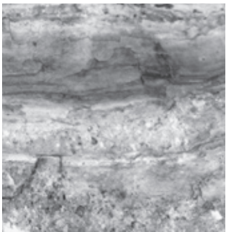
▲流紋岩
