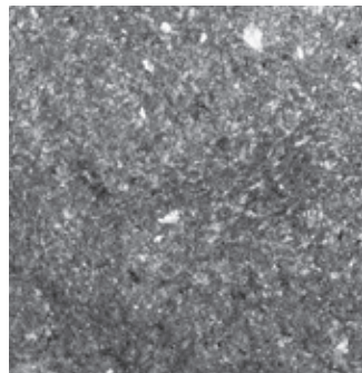
▲玄武岩
