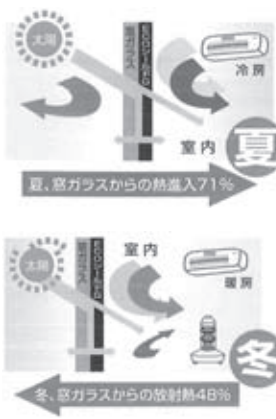
▲窓ガラスの遮熱の仕組み
