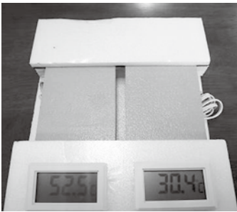
▲断熱効果実験。右の塗布済みの方が、左の塗布なしより、温度上昇が少ない
